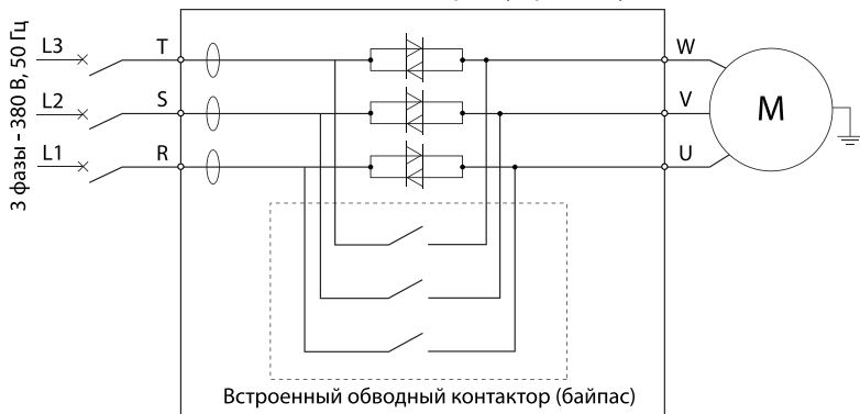
Схема подключения двигателя «в линию» для устройства плавного пуска со встроенным обводным контактором (серия SBI).
