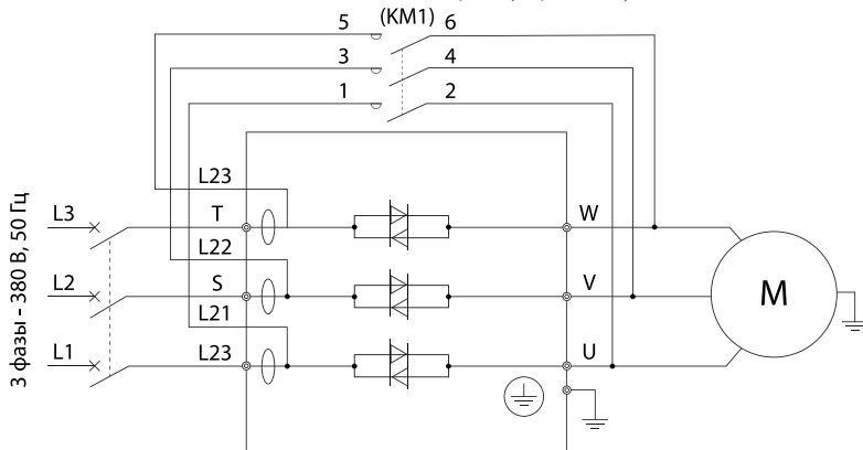
Схема подключения двигателя «в линию» для устройства плавного пуска со встроенным обводным контактором (серия SBI).
